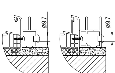
DETAIL UCHYCENÍ VODÍCÍ LIŠTY
